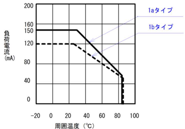
MOSFETリレー 負荷電流：周囲温度特性
